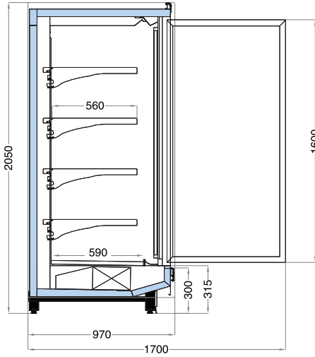
AMATIS NT 2050
