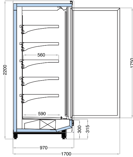
AMATIS NT 2200
