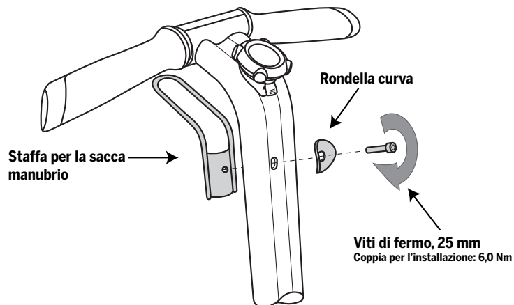
Figura 1. Installazione della staffa per la sacca manubrio
