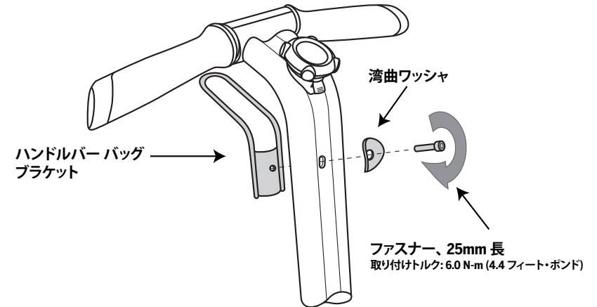
図 1. ハンドルバー バッグ ブラケットの取り付け
