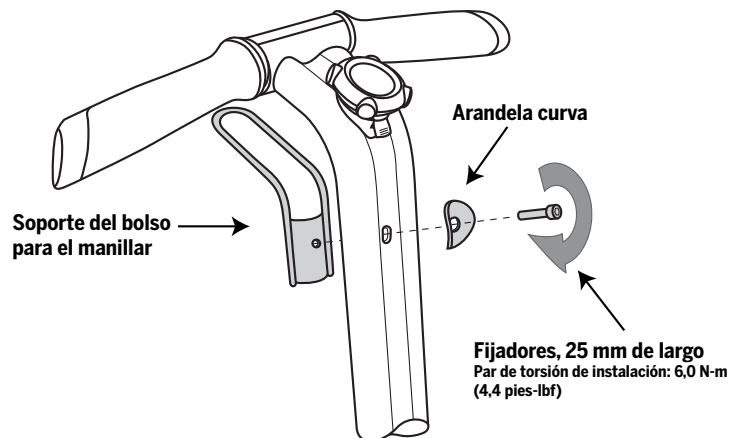
Figura 1. Cómo instalar el soporte del bolso para el manillar
