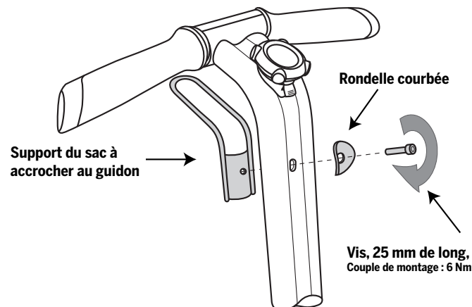
Figure 1. Installation du support du sac à accrocher au guidon
