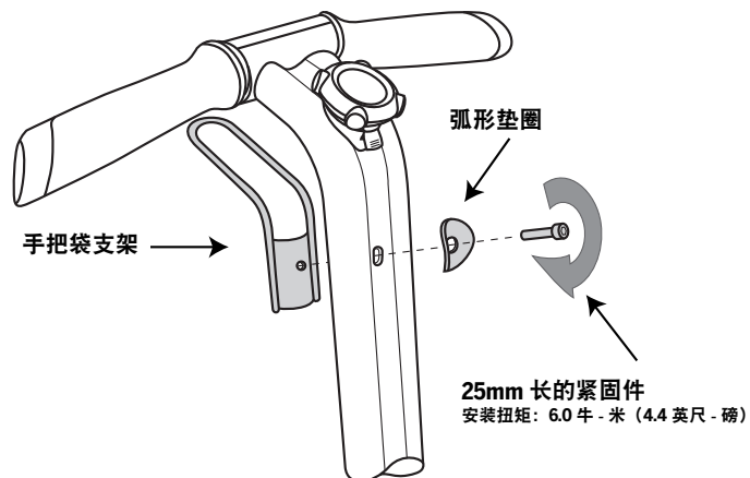
图 1. 安装手把袋支架
