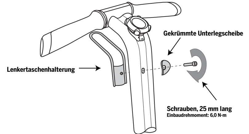
Abbildung 1. Die Lenkertaschenhalterung installieren
